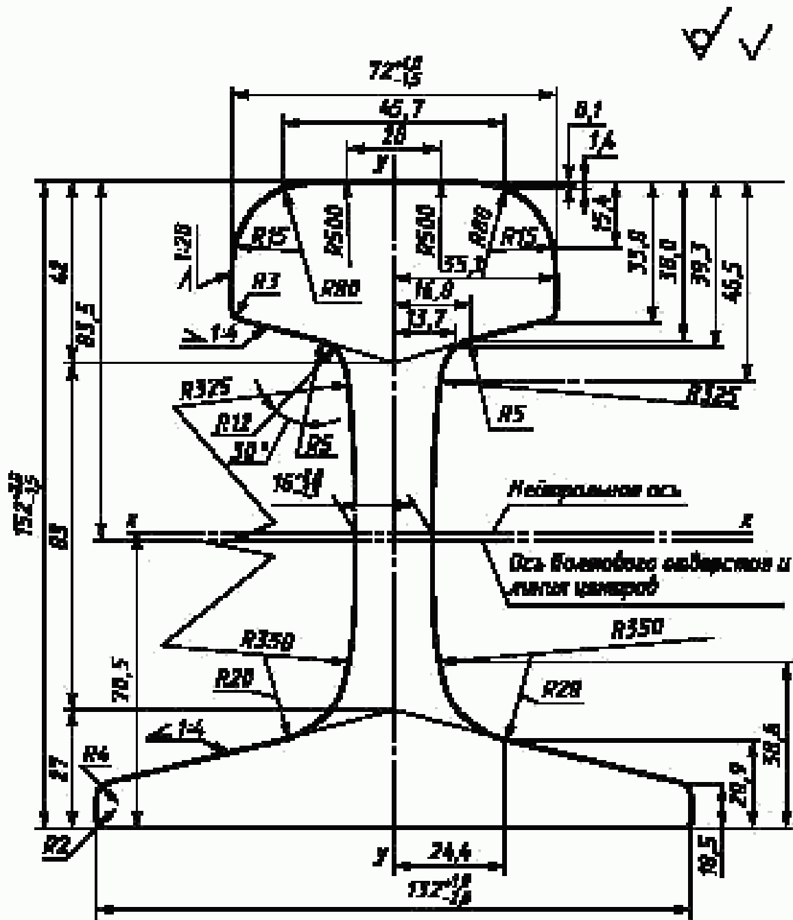
Рисунок 1 — Поперечное сечение рельса типа РП50
