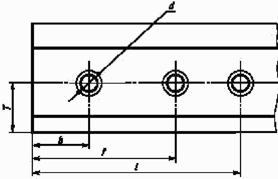
Рисунок 4 — Расположение болтовых отверстий на концах рельсов
