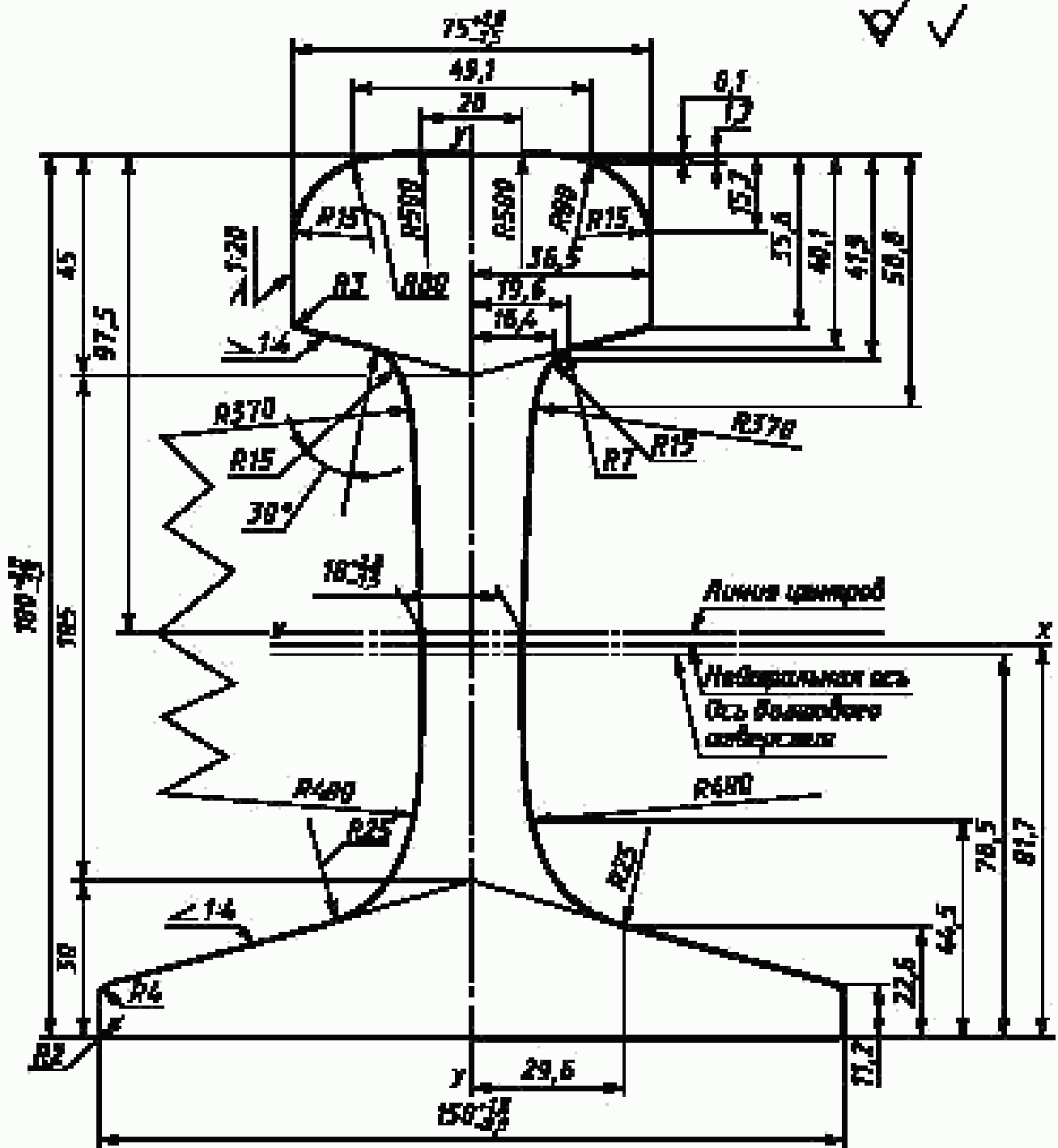
Рисунок 2 — Поперечное сечение рельса типа РП65
