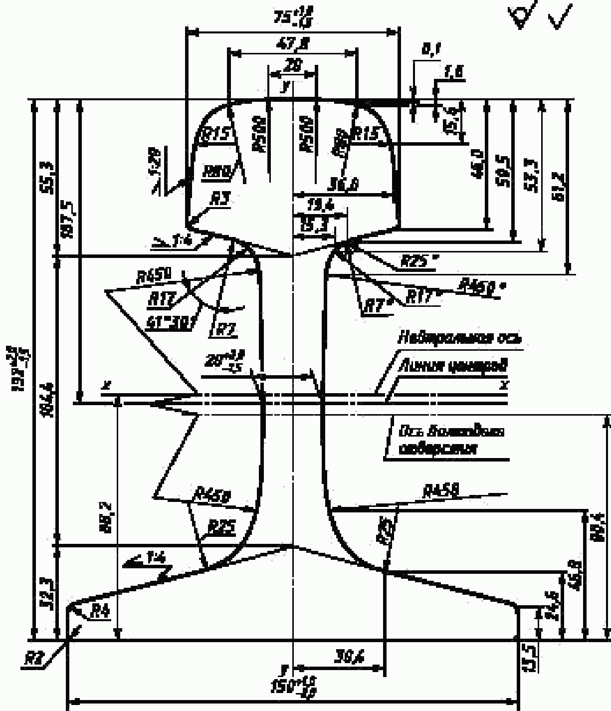
Рисунок 3 — Поперечное сечение рельса типа РП75
